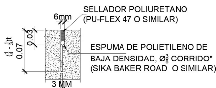
DETALLE 1
